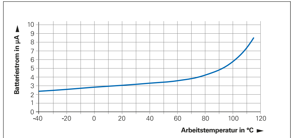
Typischer Entladestrom im Normalbetrieb ( U_{BAT} = 3,6V )
