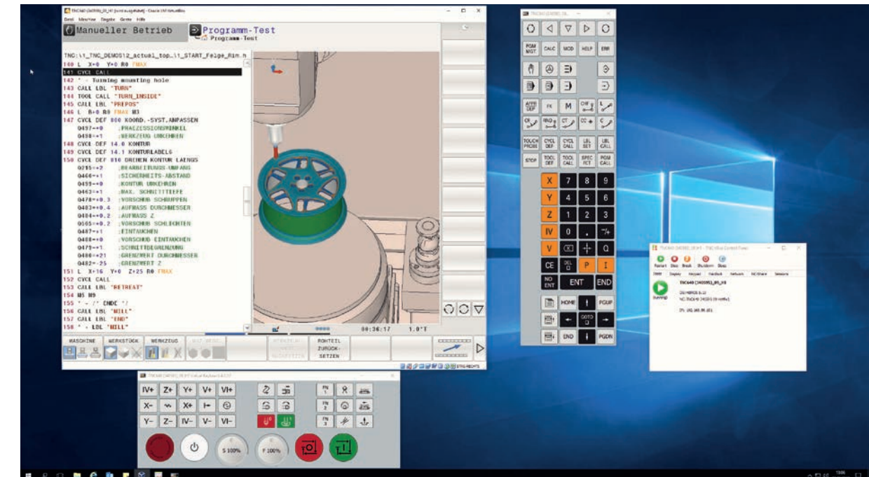
Programmierplatz mit virtuellem Keyboard
