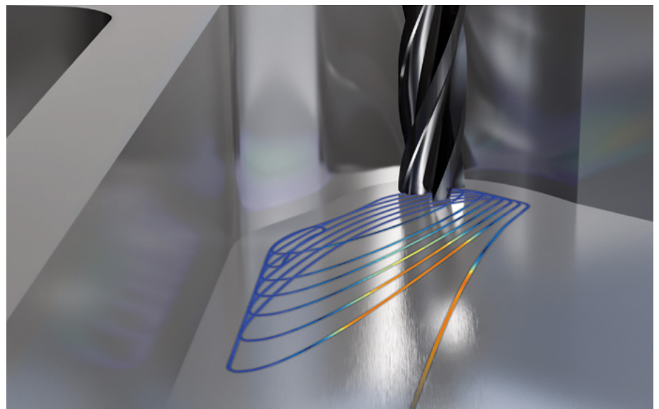
OCMを使用した加工: 6個のワーク加工後の工具
