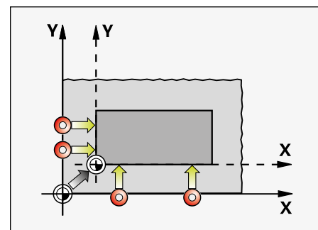
コーナー部や円柱の中心でのプリセット設定例
