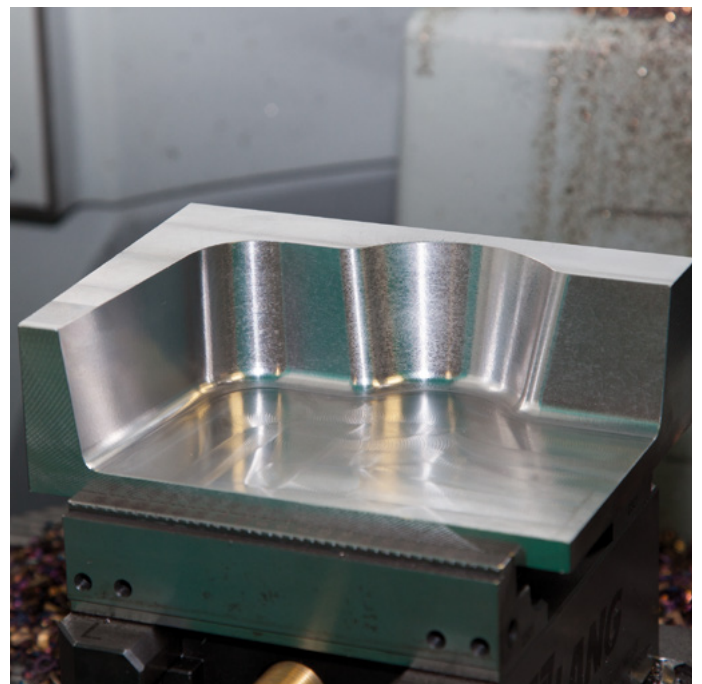
AFCにより保護された加工済みワーク
