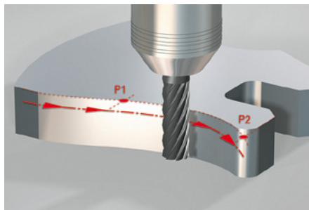
CT 終点で定義された、前の輪郭要素から途切れなく(接線方向に)接続される円弧パス
