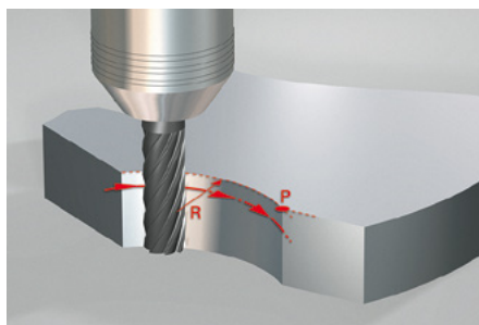
CR 半径、終点、および回転方向で定義された円弧パス
